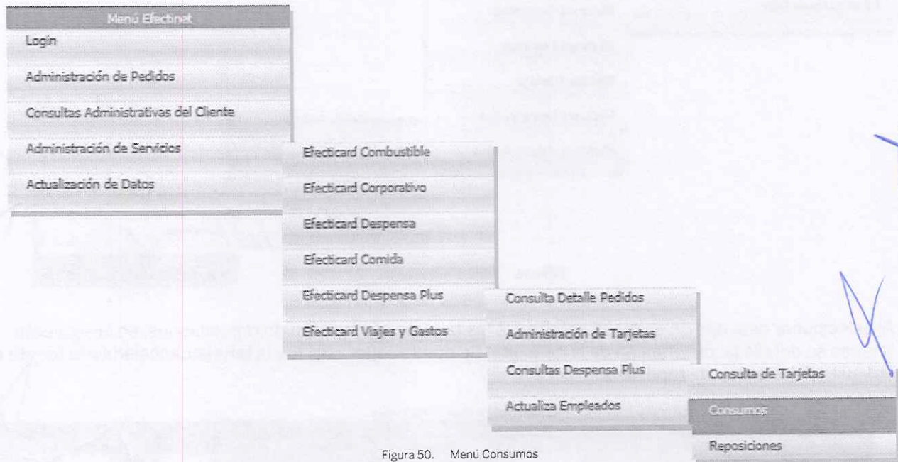
Figura 50. Menú Consumos
