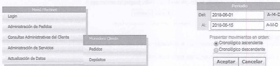
Figura 20. Monedero Cliente
